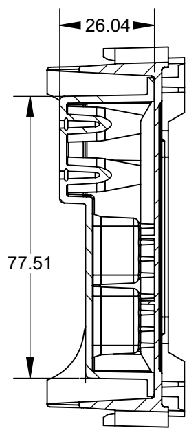
SECTION B-B SCALE: 0.7 : 1
